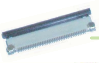
FFC Konnektör
